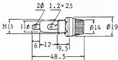
FU-1450(1A-50A)
